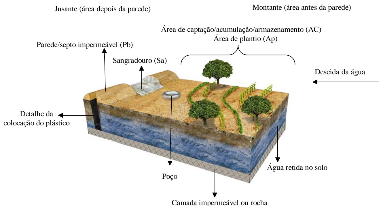
Figura 1. Desenho esquemático do funcionamento de uma barragem subterrânea com seus respectivos componentes (Desenho: Jhones Lopes).
