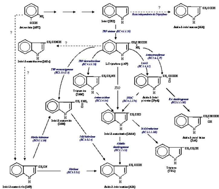
Fig. 1. Rotas e enzimas envolvidas na biossíntese de AIA em bactérias (Adaptado de PATTEN e GLICK, 1996).
