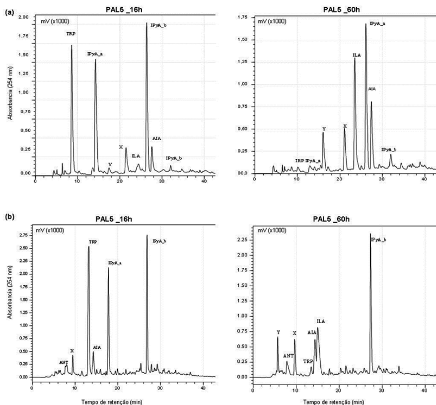
Fig. 7. Perfil cromatográfico do sobrenadante da estirpe PAL5 T após 16 e 60 horas de crescimento em meio LGI-P na presença de L-triptofano analisados por HPLC com (a) gradiente de acetonitrila:água ácida (eluyente A) ou com (b) gradiente de metanol:tampão (eluyente B) como fase móvel, após extração com o cartucho SPE-StrataX, conforme descrito na seção material e métodos. Para as abreviações verifique a Tab. 1.
