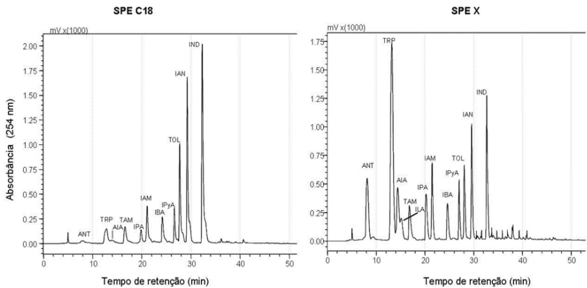
Fig. 5. Perfil cromatográfico de doze compostos indólicos analisados por HPLC com gradiente de metanol:tampão como fase móvel, após extração com os cartuchos SPE-C18 (A) e SPE-StrataX (B).
