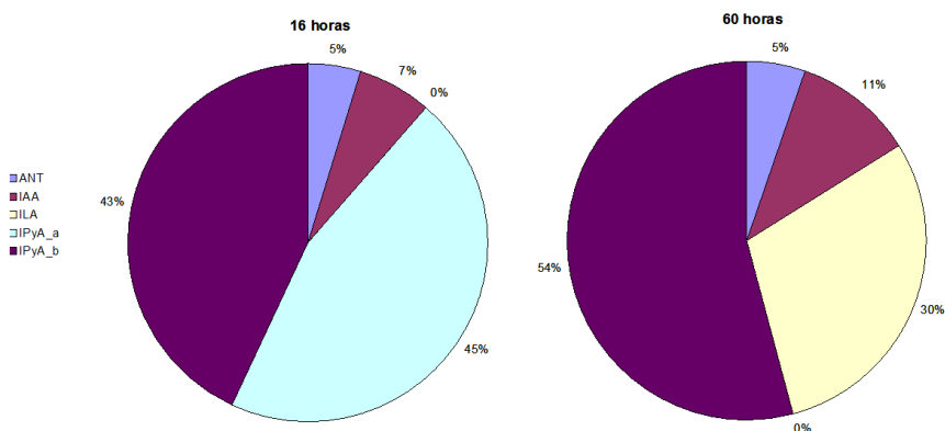
Fig. 9. Análise quantitativa por HPLC de auxinas produzidas pela estirpe selvagem de G. diazotrophicus após 16 e 60 horas de crescimento em meio de cultivo LGI-P com triptofano. Contribuição de cada composto em porcentagem para o total de compostos (conforme Tab. 4).
