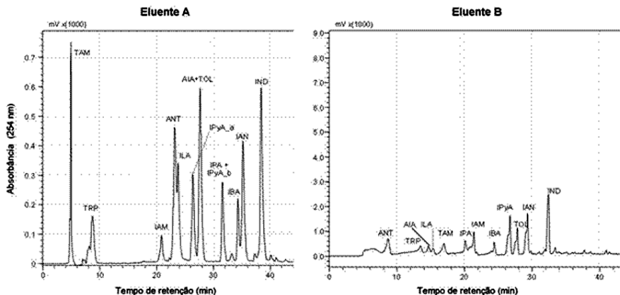
Fig. 4. Perfil cromatográfico de 12 compostos indólicos analisados por HPLC com um gradiente de acetonitrila:água ácida (Método 1) e um gradiente de metanol:tampão fosfato (Método 2) como fase móvel. Para as abreviações verifique a Tab. 1.
