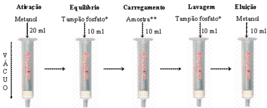
Fig. 2. Extração de compostos indólicos utilizando o sistema de extração em fase sólida (SPE). *O tampão de equilíbrio e lavagem pode ser alterado conforme o sistema de solventes utilizado. **Na análise do sobrenadante da cultura a quantidade de amostra carregada no cartucho foi 20 ml.
