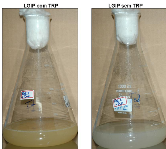
Fig. 6. Cultura de G. diazotrophicus após 60 horas de cultivo na presença e ausência de L-triptofano sob agitação (200 rpm) e 30°C.
