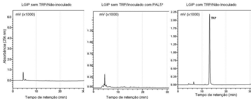
Fig. 8. Perfil cromatográfico do sobrenadante da estirpe PAL5 T na ausência de triptofano, e do meio de cultivo LGI-P (com e sem triptofano) analisados por HPLC com um gradiente de metanol: tampão (Método 2) como fase móvel, após extração com o cartucho SPE-StrataX, conforme descrito na seção material e métodos. Para as abreviações verifique a Tab. 1.
