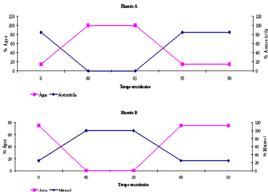
Fig. 3. Condições de análise por HPLC com o Método 1 (gradiente de acetonitrila: água MilliQ ácida pH 3,0) e com o Método 2 (gradiente de metanol:tampão fosfato pH 7,0).
