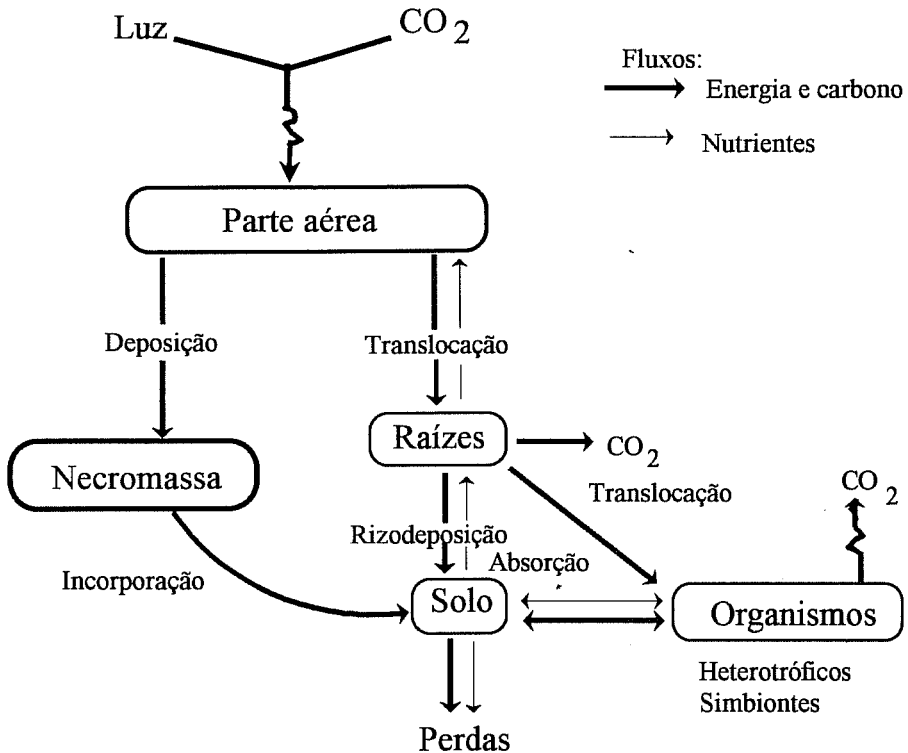
Figura 5. Fluxo de energia, carbono e nutrientes no sistema solo-planta-organismos (Siqueira 1993a).
