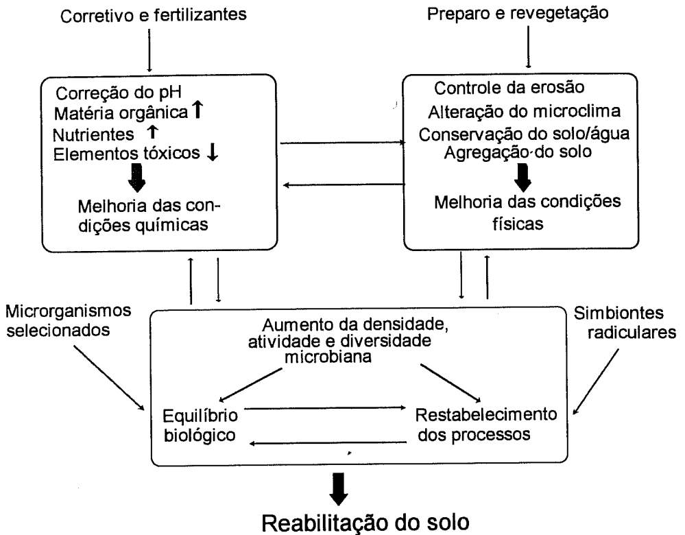
Figura 13. Principais procedimentos para reabilitação de solos degradados e as interações entre os processos físicos, químicos e biológicos.
