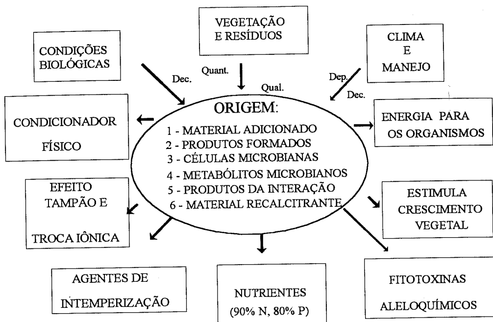
Figura 4. Origem, composição e efeitos da matéria orgânica do solo (MOS). As abreviações se referem a: Dec. (decomposição), Dep. (deposição), Quant. (quantidade), Qual. (qualidade).
