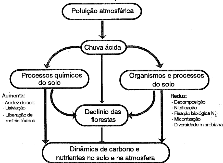
Figura 11. Impacto da poluição atmosférica sobre os processos e organismos do solo (Siqueira1993a).
