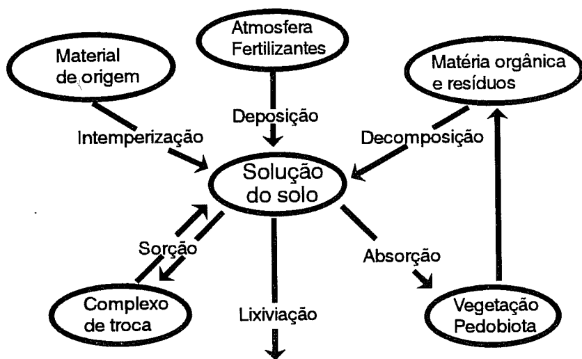
Figura 8. Compartimentalização e processos das transformações dos nutrientes no sistema solo-planta.
