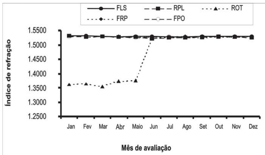
Fig. 12. Resultados médios de índice de refração de óleo essencial extraído de biomassa de pimenta longa, composta de folhas (FLS), ramos plagiográficos (RPL), ramos ortográficos (ROT), folhas e ramos finos (FRP) e folhas, ramos plagiográficos e ramos ortográficos (FPO), medido em ambiente a 25\text{ }^{\circ}\text{C} \pm 2\text{ }^{\circ}\text{C} , no período de janeiro a dezembro de 2002.
