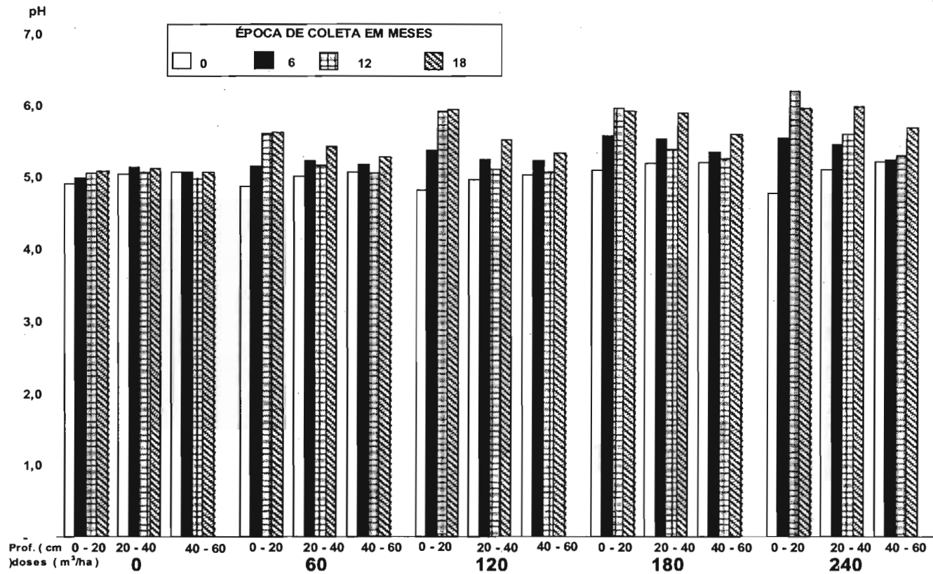
Fig.3. Efeitos de doses de efluente da agroindústria de dendê (POME) sobre o pH do solo em amostras coletadas a diferentes profundidades, após 0, 6, 12, e 18 meses de aplicações mensais.
