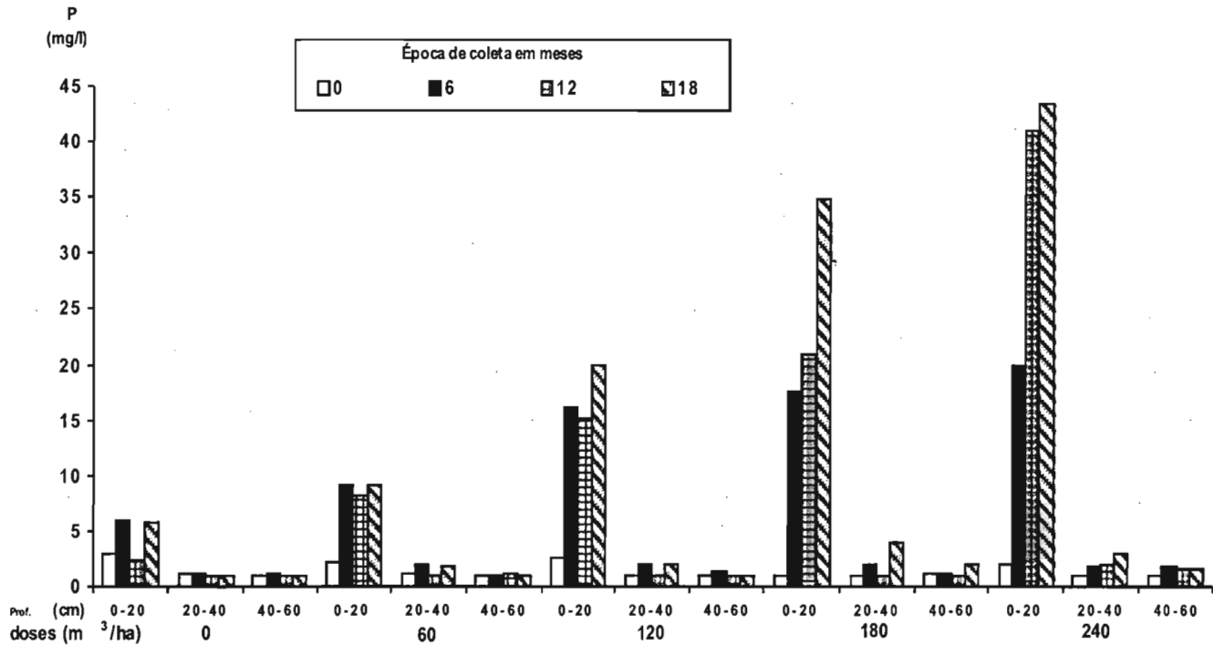
Fig.5. Efeitos de doses de efluente da agroindústria de dendê (POME) sobre o teor de P do solo em amostras coletadas a diferentes profundidades, após 0, 6, 12, e 18 meses de aplicações mensais.
