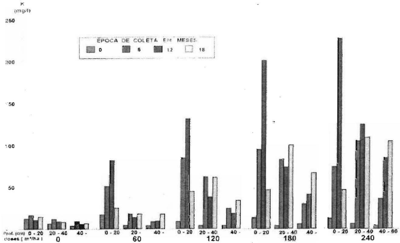
Fig.1. Efeitos de doses de efluente da agroindústria de dendê (POME) sobre o teor de K do solo em amostras coletadas a diferentes profundidades, após 0, 6, 12, e 18 meses de aplicações mensais.
