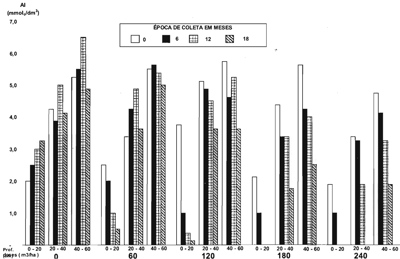
Fig.4. Efeitos de doses de efluente da agroindústria de dendê (POME) sobre o teor de Al do solo em amostras coletadas a diferentes profundidades, após 0, 6, 12, e 18 meses de aplicações mensais.
