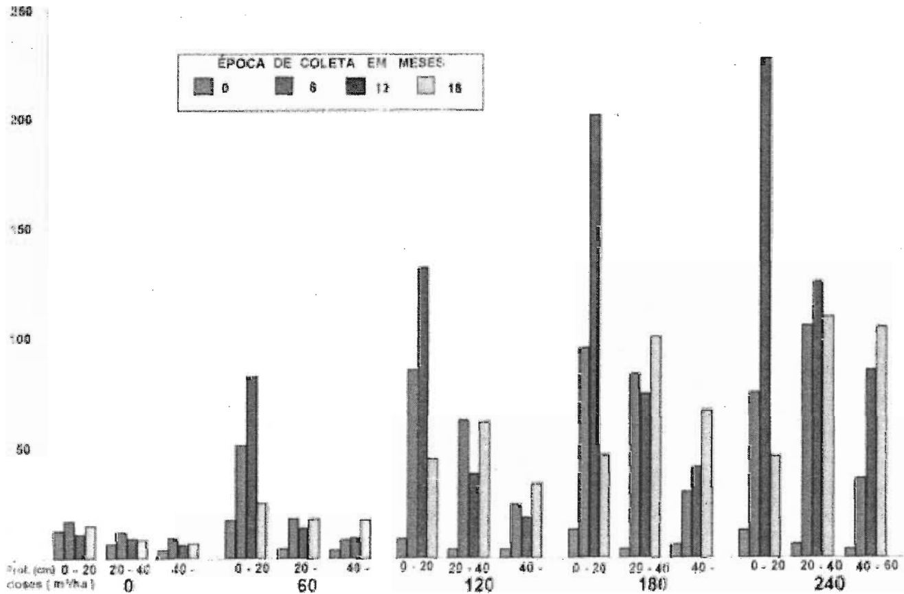
Fig.2. Efeitos de doses de efluente da agroindústria de dendê (POME) sobre o teor de Ca + Mg do solo em amostras coletadas a diferentes profundidades, após 0, 6, 12, e 18 meses de aplicações mensais.
