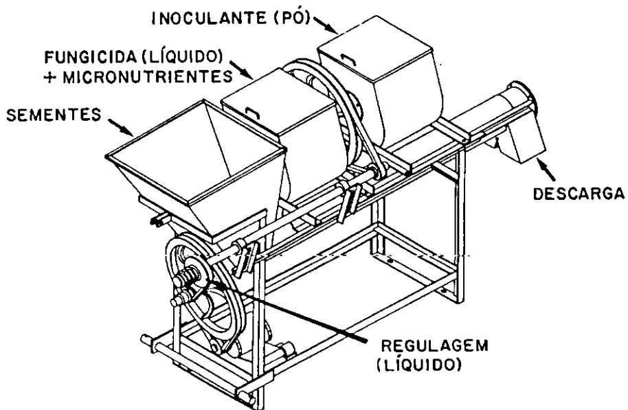
FIG. 3. Máquina de tratar sementes (Adaptado de Grazmec).
