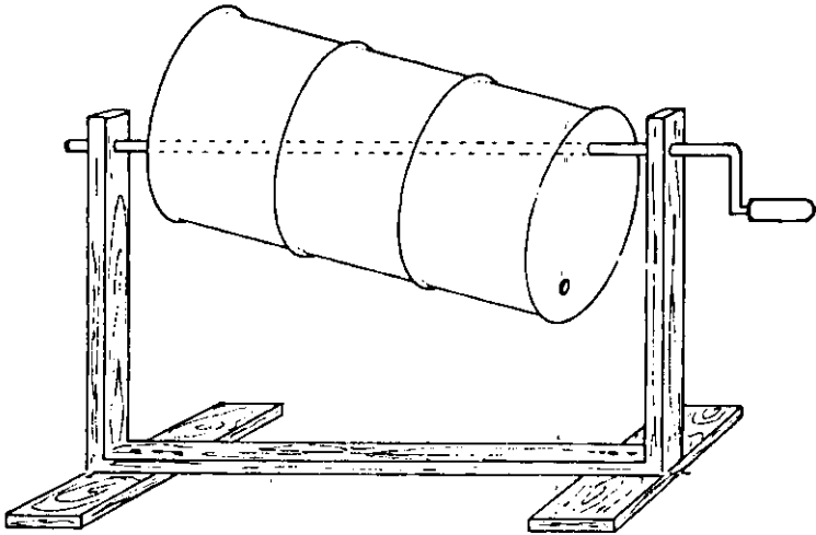
FIG. 4. Tambor giratório com eixo excêntrico para tratar sementes.
