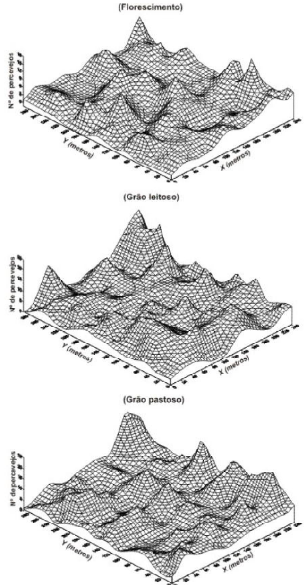
Fig. 4. Distribuição espacial de Oebalus spp. em campos de arroz irrigado
