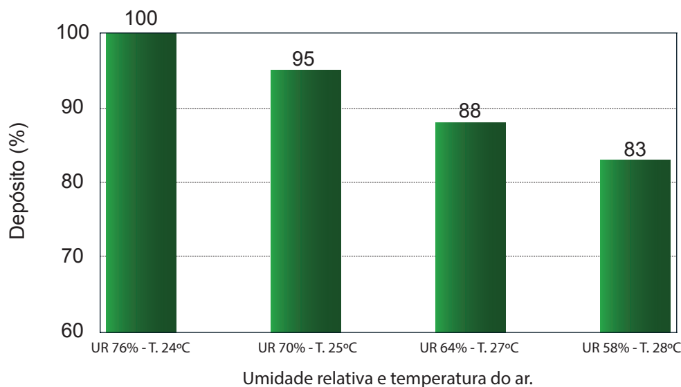
Figura 5. Depósitos porcentuais de pulverização sobre folhas de maçã em diferentes condições ambientais no momento da aplicação.
