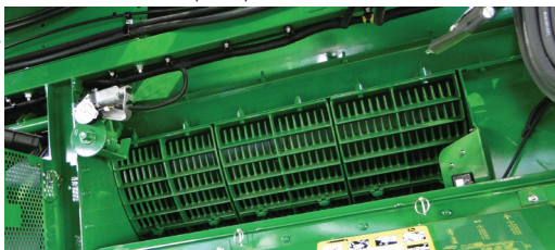
Figura 1. Sistema tangencial de trilha presente em máquinas colhedoras, mostrando o cilindro batedor e côncavo.
