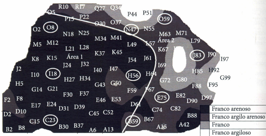
Figura 4. Especialização da textura do solo, zonas homogêneas e indicação das plantas avaliadas e dos locais de monitoramento da umidade do solo em pomar de pessegueiro (Fonte: TERRA, 2012).
