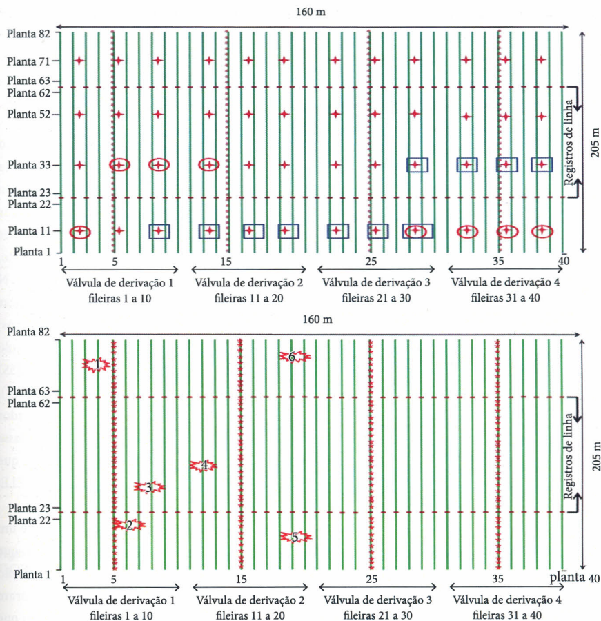
Figura 1. Pontos de coleta de amostras de solo a 0-0,2 m e 0,2-0,4 m (fileiras 5, 15, 25 e 35) e pontos de trradagem até 1,0 m de profundidade (cruz vermelha). Círculos vermelhos e retângulos azuis representam, respectivamente, presença de concreções entre 0,6 e 1,0 m e solo encharcado entre 0,6 e 1,0 m (superior). Os pontos de monitoramento de umidade do solo, em cada uma das seis zonas de manejo determinadas, nas duas válvulas de irrigação (inferior).
