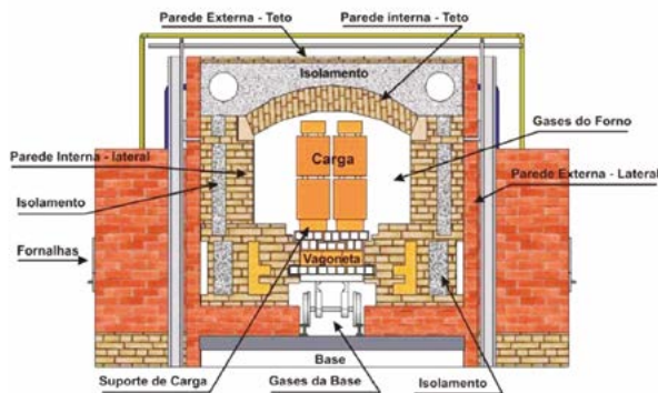
Figura 8.15 – Ilustração da seção transversal de um forno túnel.
