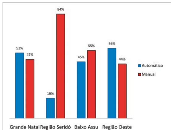
Figura 7.10 – Relação percentual de caixões alimentadores automáticos e manuais das cerâmicas do RN.
