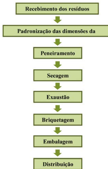
Figura 10.10 – Fluxograma do processo de produção de briquetes.
