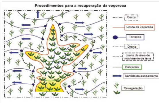
Figura 6.114 – Esquema representativo dos procedimentos para a recuperação de voçoroca.
