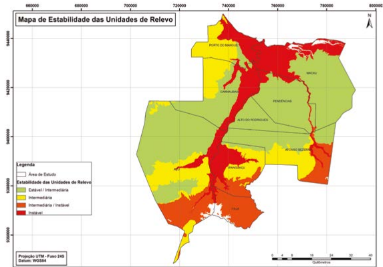
Figura 5.3 – Mapa de estabilidade das unidades de relevo.
